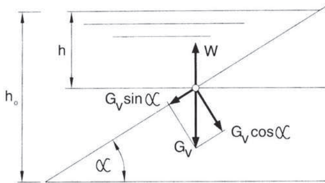
Rys. 2. Schemat działania sił na cząstkę materiału w wodzie – G_V jest siłą ciężkości w wodzie [1]
