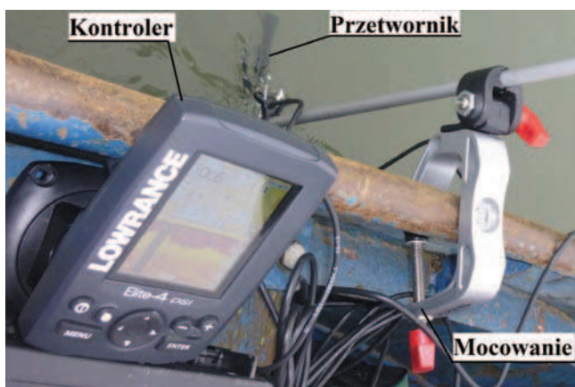
Rys. 4. Sonda akustyczna Lowrance Elite-4 DSI wykorzystana w pomiarach batymetrycznych (Fot. D. Madusiok)
