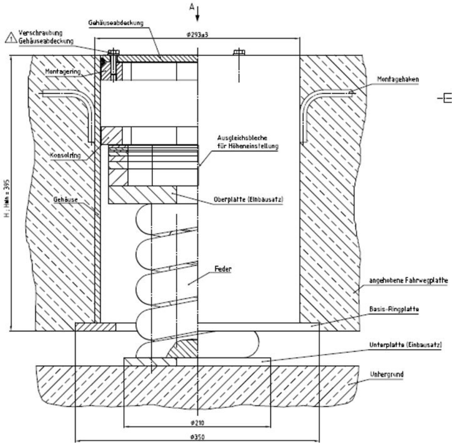
Rys. 7. Budowa wibroizolatora typu GSI {3}
