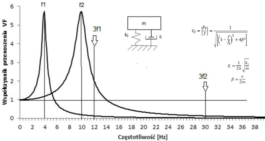
Rys. 1. Zasada wibroizolacji
