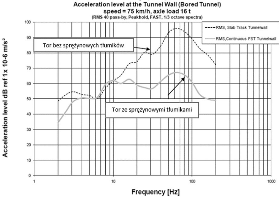
Rys 14. Zestawienie wartości poziomu drgań zarejestrowanych na ścianie tunelu w punkcie H1 dla nawierzchni tunelu z płytą betonową bez wibroizolatorów sprężynowych i nawierzchni tunelu z wibroizolatorami sprężynowymi {2}
