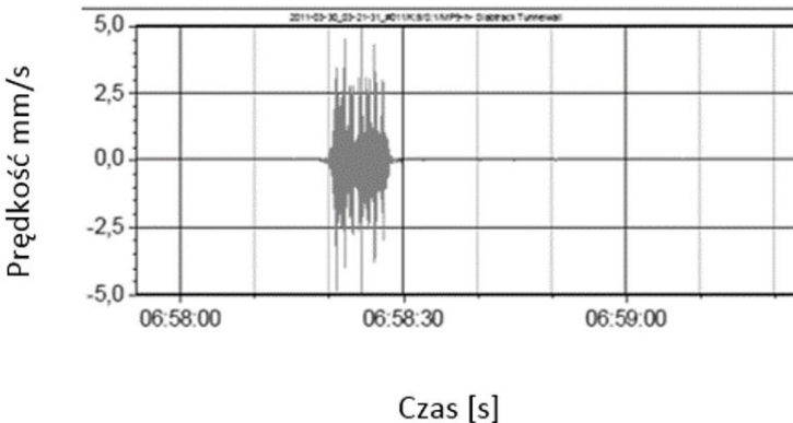
Rys. 13. Przykładowe wyniki pomiaru prędkości drgań w funkcji czasu dla czujników zlokalizowanych na ścianach tunelu metra - nawierzchnia bez tłumików sprężynowych {2}
