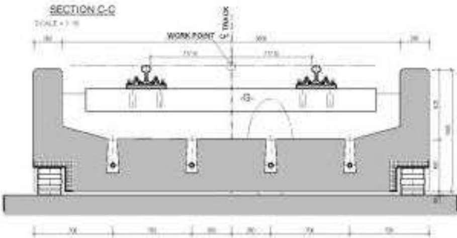
Rys. 5b. Wibroizolatory KY w podsypkowej nawierzchni szynowej {3}
