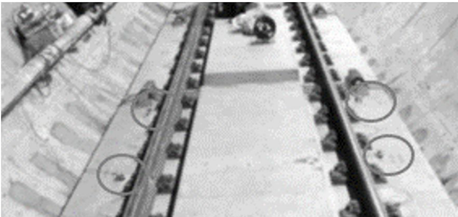
Rys. 11. Lokalizacja czujników pomiarowych na płycie betonowej z systemem wibroizolacji sprężynowej na linii metra nr 10 w Szanghaju {1}
