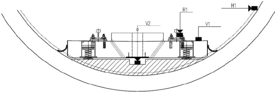
Rys. 10. Schemat nawierzchni bezpodsypkowej z wibroizolacją sprężynową wraz z zaznaczonymi punktami pomiarowymi V2, R1, V1, H1 {2}
