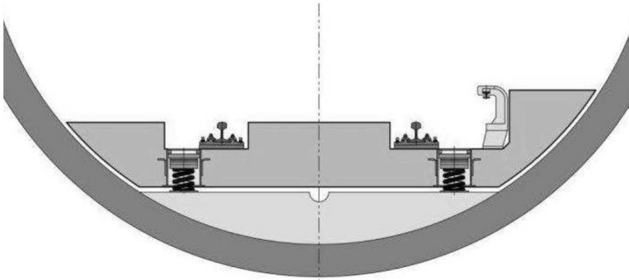
Rys. 3. Wibroizolatory GSI w bezpodsypkowej nawierzchni szynowej w tunelu [3]
