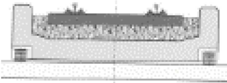
Rys. 5a. Wibroizolatory KY w podsypkowej nawierzchni szynowej {3}
