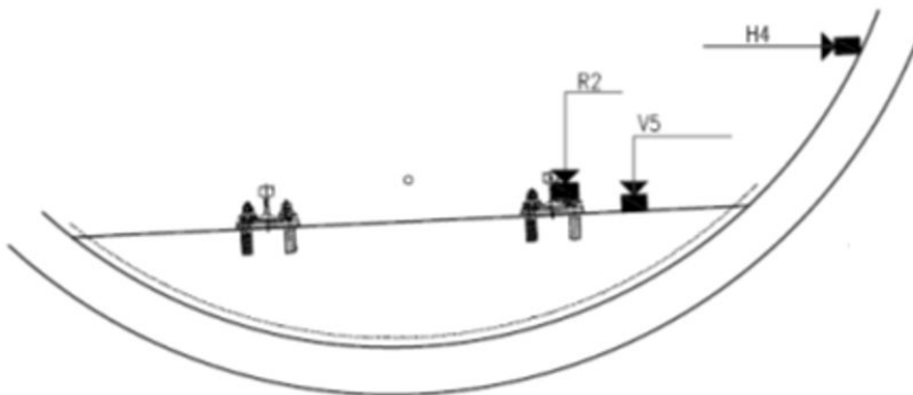
Rys. 9. Schemat nawierzchni bezpodsypkowej bez sprężyn wraz z zaznaczonymi punktami pomiarowymi V2, R1, V1, H1 {2}
