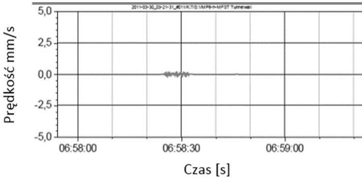
Rys. 12. Przykładowe wyniki pomiaru prędkości rejestrowanego sygnału w funkcji czasu dla czujników zlokalizowanych na ścianach tunelu metra - nawierzchnia z tłumikami sprężynowymi {2}
