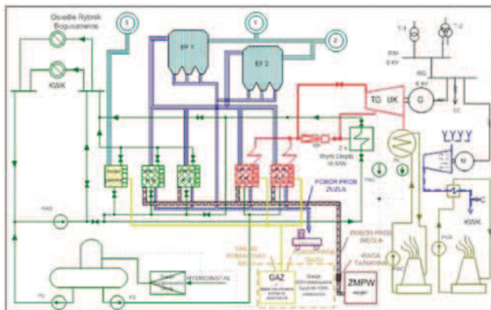
Rys. 10. Schemat Elektrociepłowni Jankowice w Zakładzie Elektrociepłowni
