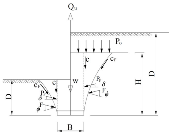
Rys. 1. Schemat pracy fundamentu przy wyciąganiu wg Meyerhoffa [6]
