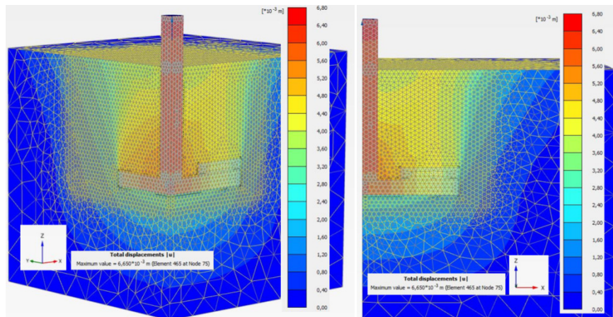
Rys. 7. Mapy deformacji dla fazy zniszczenia modelu MES
