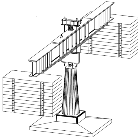
Rys. 3. Schemat aksonometryczny stanowiska badawczego Pilettest [8]
