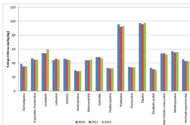
Rys. 4. Emisja CH_4 w Polsce w układzie terytorialnym w latach 2010-2012 w przeliczeniu na jednego mieszkańca [GUS 2015]
