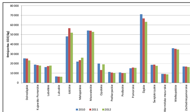
Rys. 7. Łączna emisja GHG w Polsce w układzie terytorialnym w latach 2010-2012 wyrażona w ekwiwalencie CO 2 [GUS 2015]
