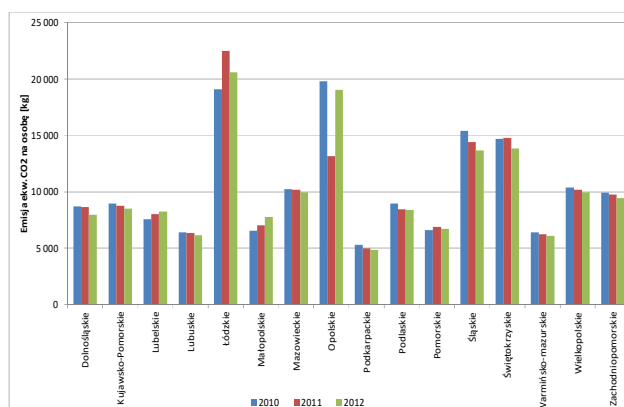
Rys. 8. Łączna emisja GHG w Polsce w układzie terytorialnym w latach 2010-2012 wyrażona w ekwiwalencie CO 2 i w przeliczeniu na jednego mieszkańca [GUS 2015]
