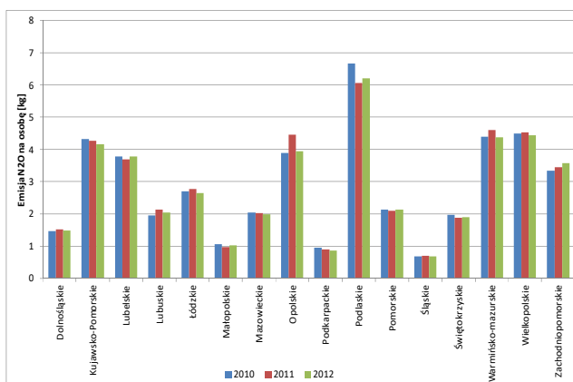
Rys.6. Emisja N_2O w Polsce w układzie terytorialnym w latach 2010-2012 w przeliczeniu na jednego mieszkańca [GUS 2015] Fig. 6. Emissions of N_2O in Poland in a territorial for the 2010-2012 period per capita [GUS 2015]
