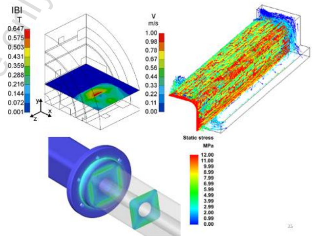
Rys. 13. Przykładowe rozkłady przestrzenne pól magnetycznych, pola prędkości płynu magnetorologicznego oraz naprężeń mechanicznych w liniowo-obrotowym hamulcu magnetorologicznym
