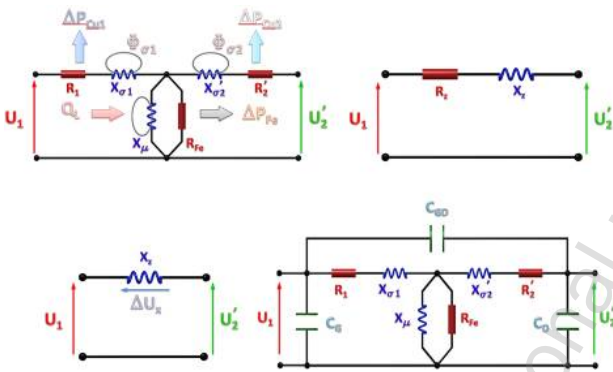
Rys. 41. Zestawienie różnych schematów zastępczych transformatora
