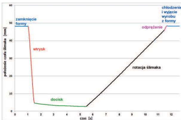
Rys. 11. Położenie czoła ślimaka podczas wtryskiwania PP z zaznaczonymi etapami cyklu wtryskowego ( T_b=230 °C, pp=10 MPa, tp=20 s, v=240 obr/min)
