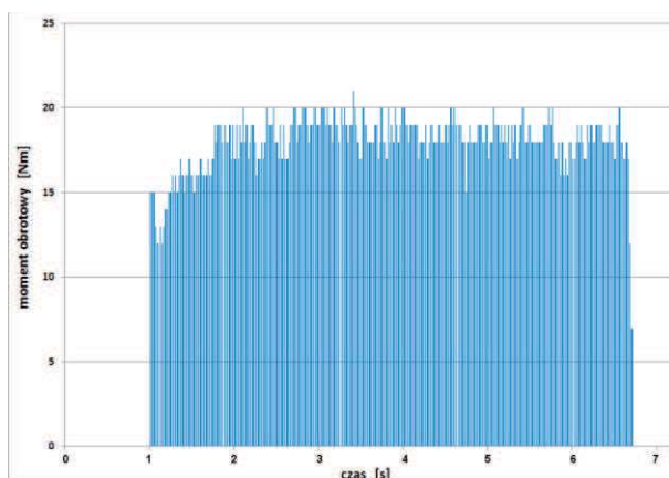
Rys. 12. Moment obrotowy ślimaka w trakcie rotacji ślimaka podczas wtryskiwania PP ( T_b=230 °C, pp=10 MPa, tp=20 s, v=240 obr/min)
