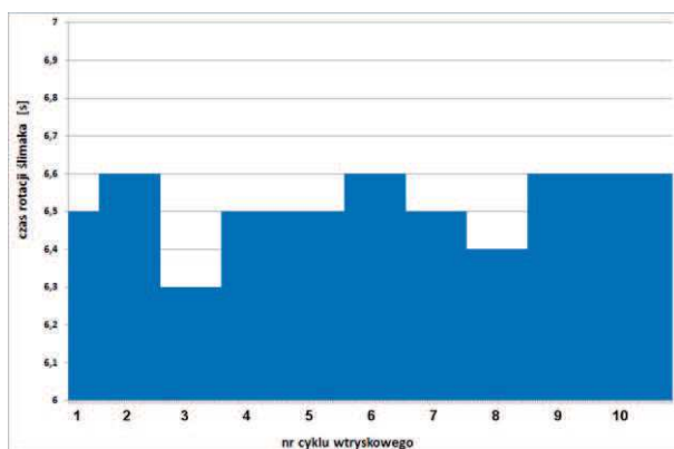
Rys. 13. Czas rotacji ślimaka w kolejnych cyklach wtryskiwania PP ( T_b=230 °C, pp=10 MPa, tp=20 s, v=240 obr/min)
