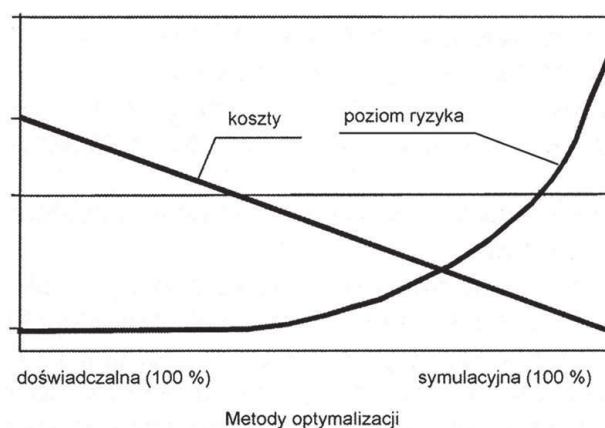
Rys. 1. Poglądowa zależność kosztów optymalizacji oraz ryzyka konstrukcyjnego ślimaka wytłaczarskiego od zastosowanej metody optymalizacji [2]
