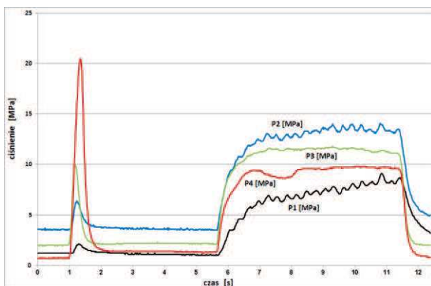
Rys. 10. Ciśnienie tworzywa w cylindrze (jeden cykl wtryskowy) podczas wtryskiwania PP ( T_b=230 °C, pp=10 MPa, tp=20 s, v=240 obr/min)
