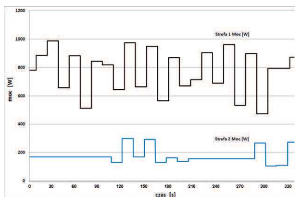
Rys. 14. Pobór mocy przez grzałki podczas wtryskiwania PP ( T_p=230\text{ }^\circ\text{C} , p_p=10\text{ MPa} , t_p=20\text{ s} , v=240\text{ obr/min} )
