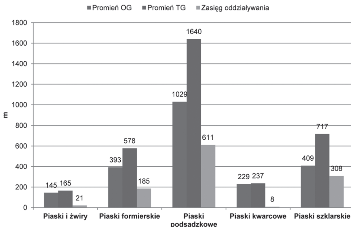
Rys. 2. Przybliżone zasięgi oddziaływania robót górniczych
