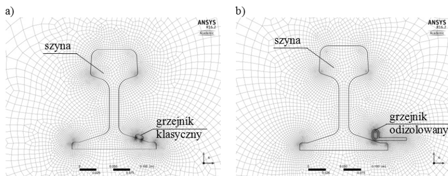
Rys. 2. Siatka elementów skończonych w analizie 2D dla układu z grzejnikiem: a) klasycznym, b) odizolowanym od stopki szyny
