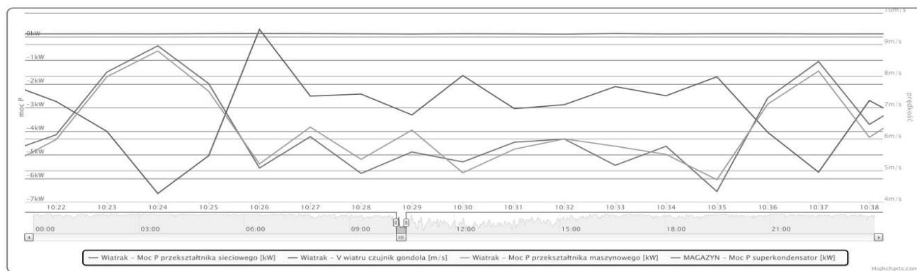
Rys. 8. Przebiegi mocy przekształtnika maszynowego, sieciowego i prędkości wiatru zarejestrowane przez system ECV-2.0
