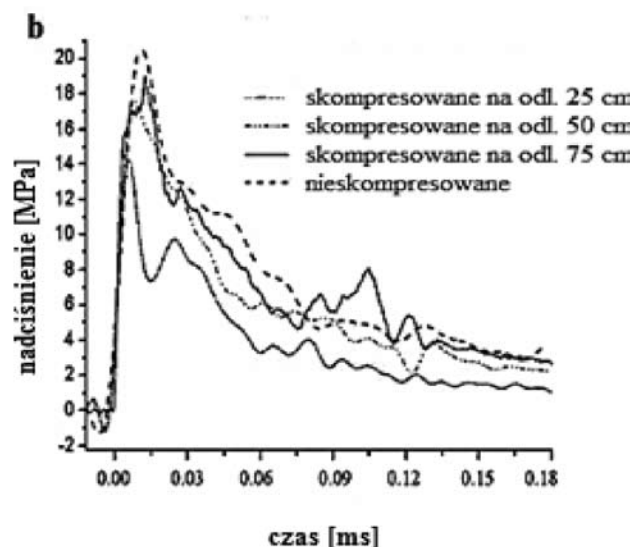
Rys. 11. Przebiegi krzywych nadciśnienia w czasie dla MWE uczulonych: a) szkłami mikrosferami, b) \text{H}_2\text{Mg} [16]
