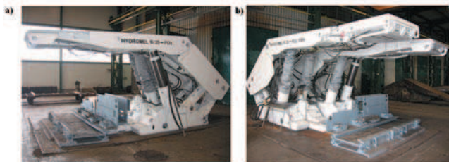
Rys. 3. Obudowa zmechanizowana HYDROMEL-16/35-POz (a) – oraz HYDROMEL-16/35-POz/BSN (b)
