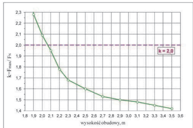
Rys. 4. Przewidywane przeciążenie stojaka obudów zmechanizowanych HYDROMEL-16/35-POz i HYDROMEL-16/35-POz/BSN w warunkach ściany 152 pokład 510 dla zaworów z układem hydraulicznym o wydajności 650 l/min
