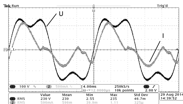
Rys. 8. Oscylogram prądu obciążenia I lampy SOX oraz napięcia zasilającego U . Próba 101 – napięcie zasilające: 30% udział 3. harmonicznej o fazy początkowej \alpha = 0^\circ
