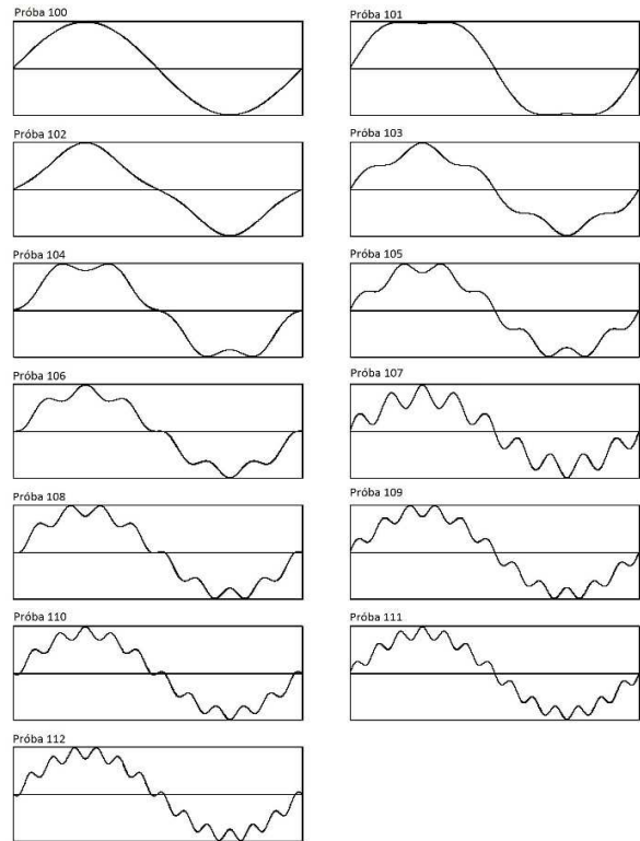
Rys. 2. Napięcia wyjściowe zasilacza programowanego dla ustawień zawartości harmonicznych zgodnie z tabelicą 1
