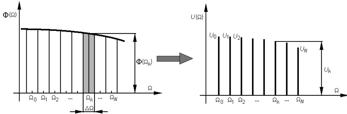
Fig. 6. Discretization of the power spectral density Fig. 6. Discrétisation du spectre de la densité de puissance
