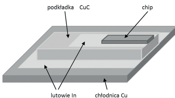
Rys. 1. Chip laserowy przyłutowany do podkładki CuC i chłodnicy Cu.
