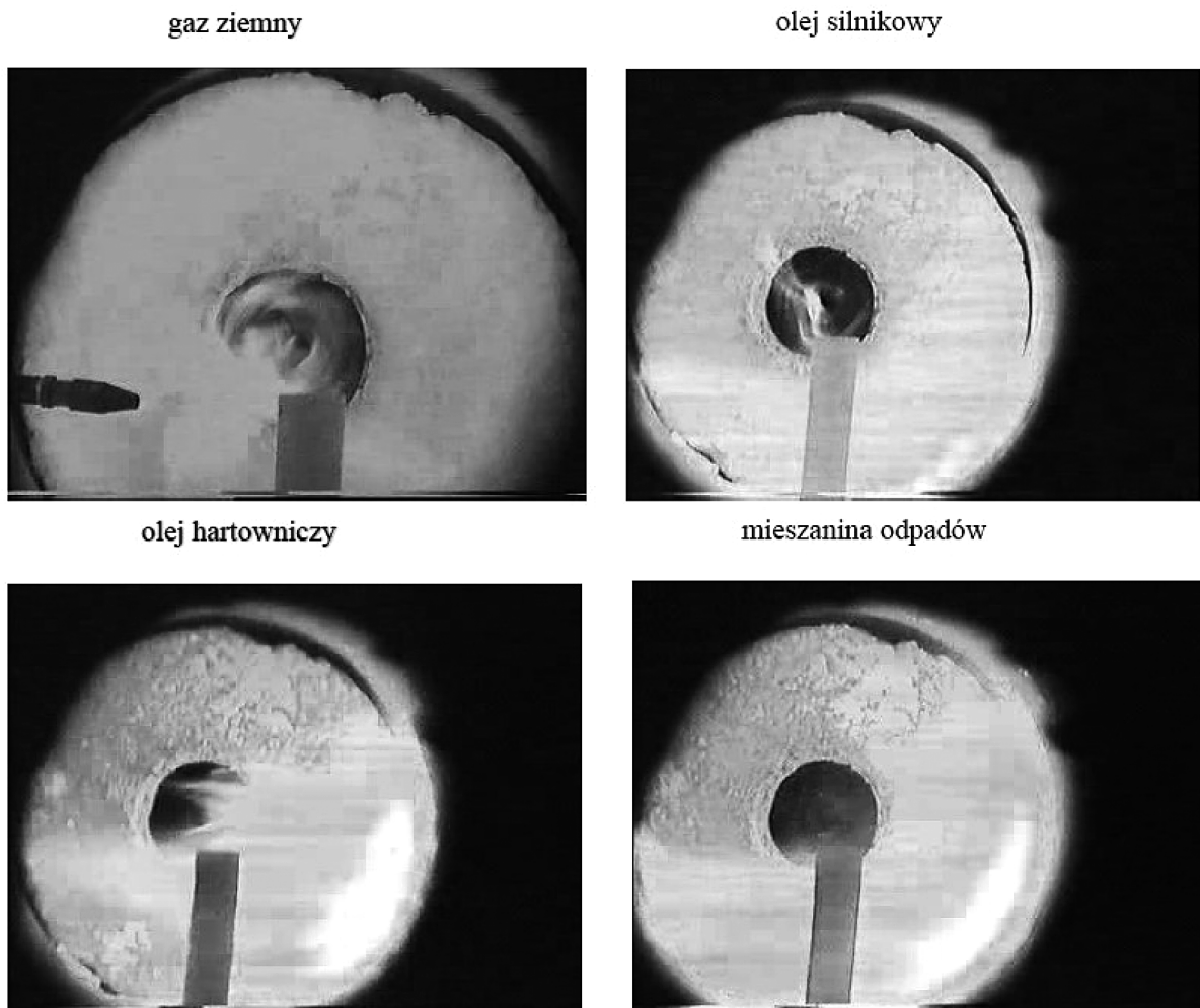
Rysunek 7 Wizualizacja procesu spalania
