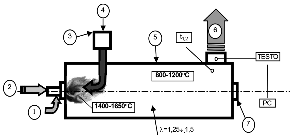
Rysunek 1 Schemat stanowiska do spalania odpadów ciekłych w komorze z wykorzystaniem palnika gazowego
