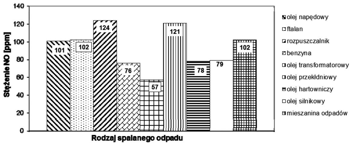
Rysunek 6 Średnie wartości stężeń NO przy statycznych parametrach wejściowych
