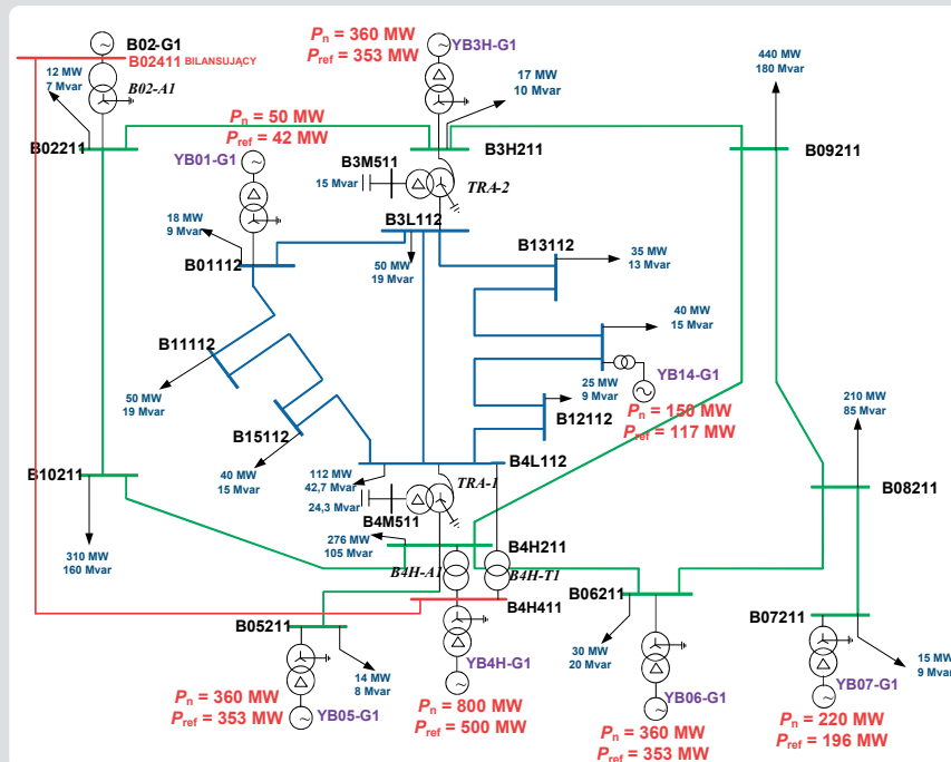
Rys. 1. Schemat systemu CIGRE wykorzystany w badaniach
