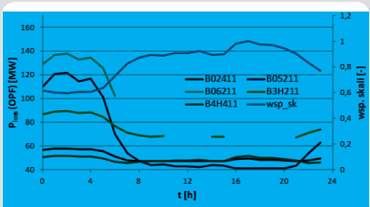
Rys. 10. Straty mocy w sieci. Zmiana lokalizacji generatora bilansującego. Z optymalizacją (OPF)
