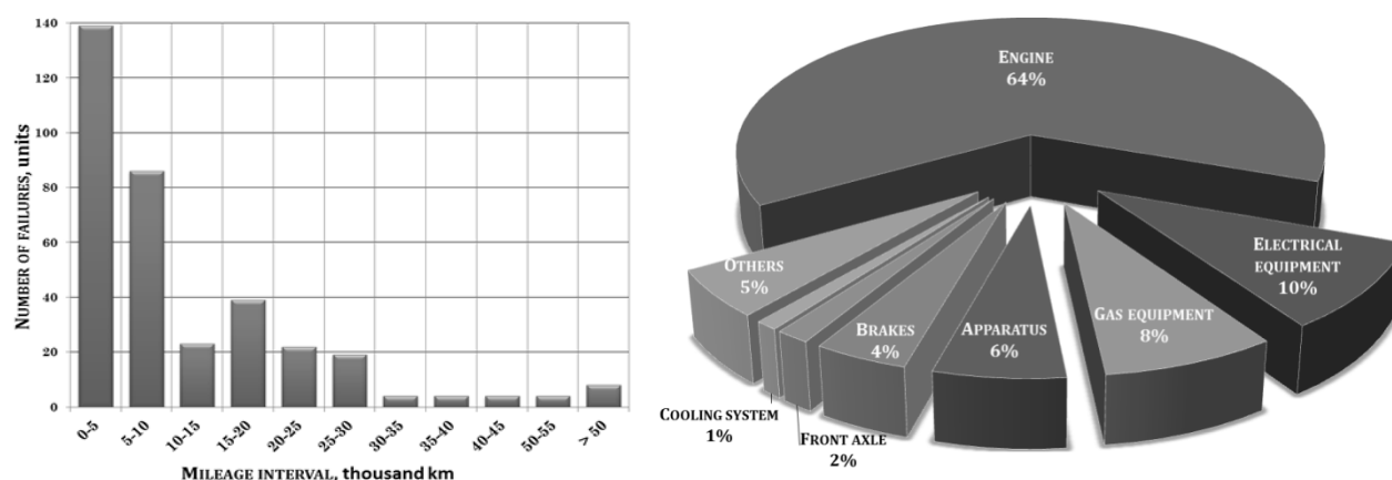
Fig. 12. Failure statistics: a) dependence on mileage; b) place of origin Рис. 12. Статистика отказов: а) зависимость от пробега; б) по месту возникновения
