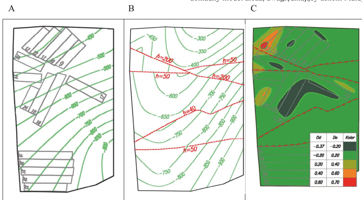
Rys. 2. Model złoża; A - uproszczony, B - dokładny, C - różnice w obliczeniach (źródło: opracowanie własne) Fig. 2. Deposit model; A - simplified, B - precise, C - differences in calculations (source: own elaboration)
