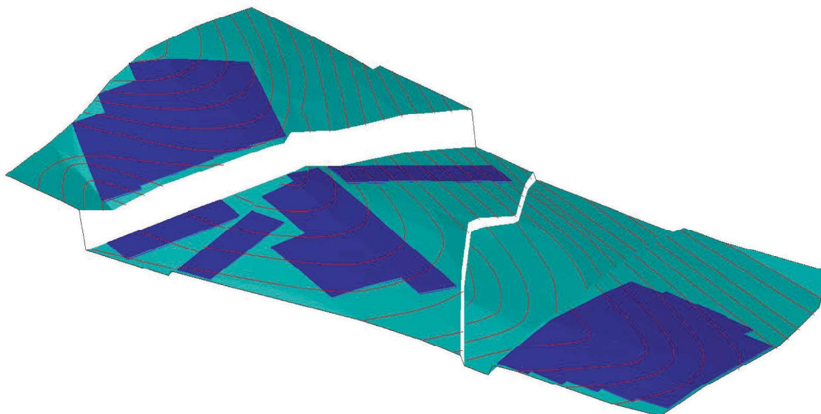
Rys. 1. Wprowadzenie uskoków i fałdów do pokładu (źródło: opracowanie własne) Fig. 1. The introduction of faults and folds to the seam (source: own elaboration)
