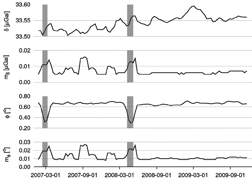
Fig. 9. Tidal parameters for M2 constituent.
