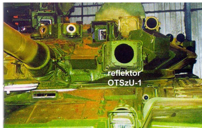
Rys. 13. Wieża czołgu T-90 z reflektorem OTSzU-1 (fot. Siergiej Suworow) [5]
