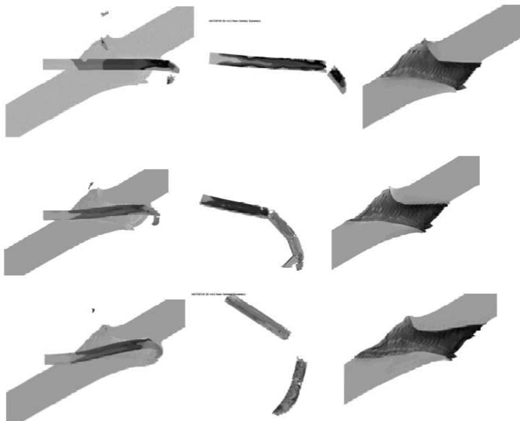
Rys.11. Wyniki symulacji dla kątów podejścia pocisku do płyty – od góry 0^\circ , 1^\circ , 2,4^\circ [7]
