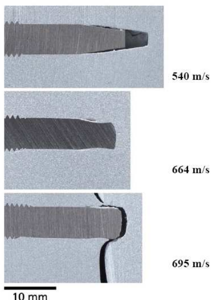
Rys. 6. Identyfikacja zjawiska uplastycznienia się czoła penetratora podczas procesu penetracji stopu 7020 wraz ze wzrostem prędkości uderzenia [4]
