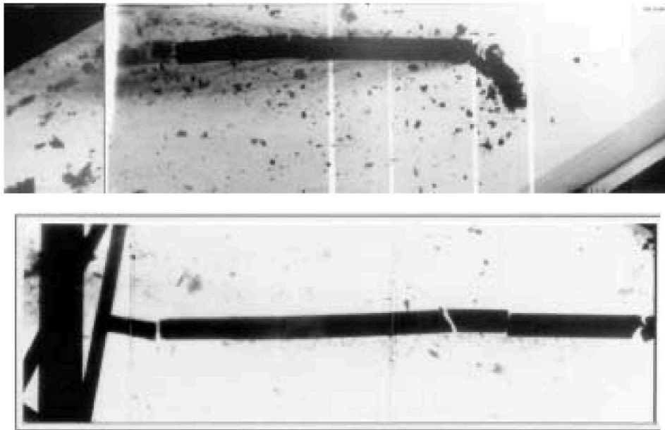
Rys.12. Wyniki badania penetracji pancerza warstwowego dla penetratorów l/d=20 (u góry) i l/d=30 (u dołu) [8]
