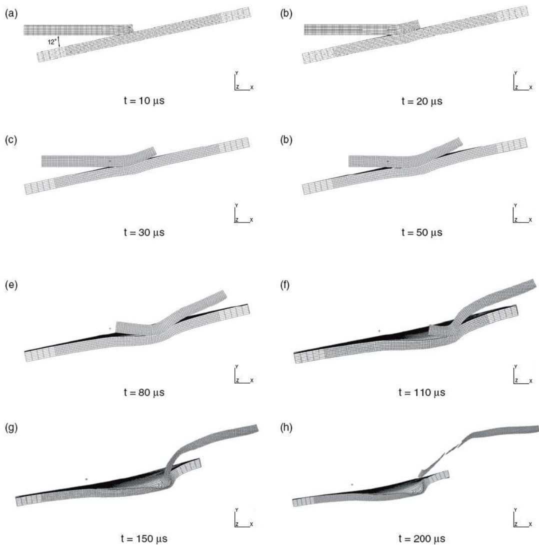
Rys. 2. Wyniki symulacji dla prędkości uderzenia 1000 m/s i kąta pochylenia płyty RHA równego 12^\circ [2]
