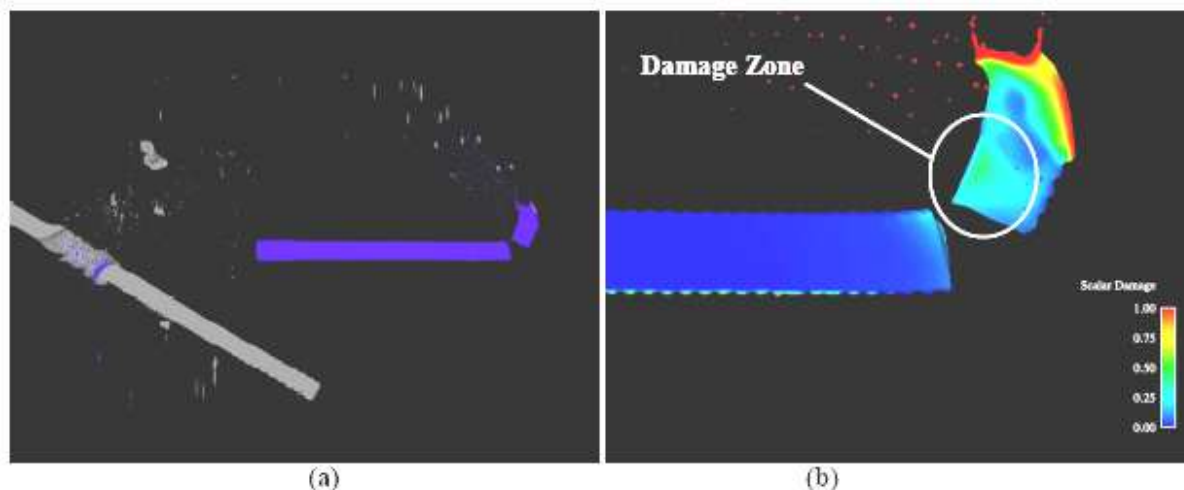
Rys. 7. Numeryczna analiza niszczenia czoła penetratora podczas zderzenia z pochyloną płytą [5]
