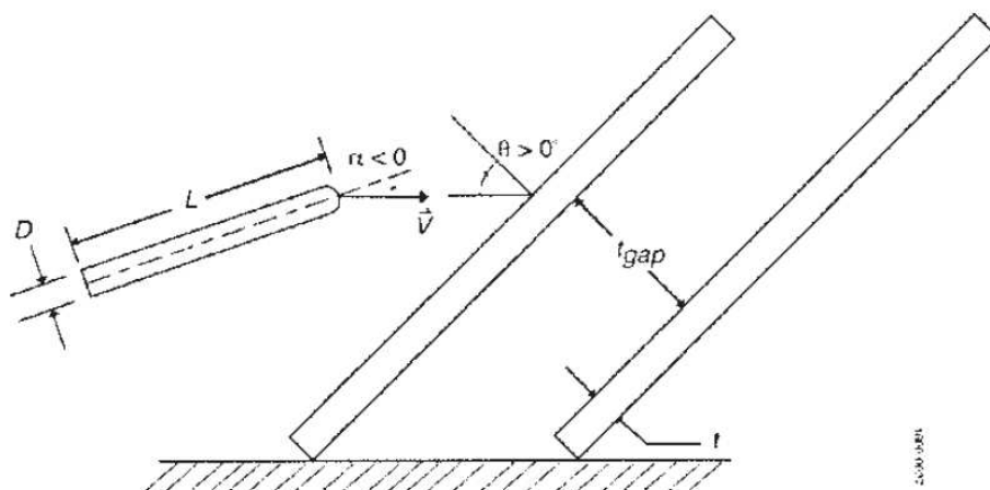
Rys. 9. Zasymulowany w pracy [6] układ badawczy
