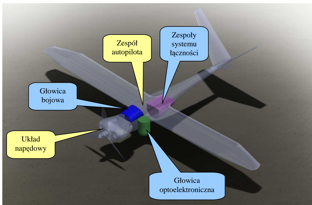
Rysunek 2.7. Rozmieszczenie w płatowcu zespołów wyposażenia BSU
