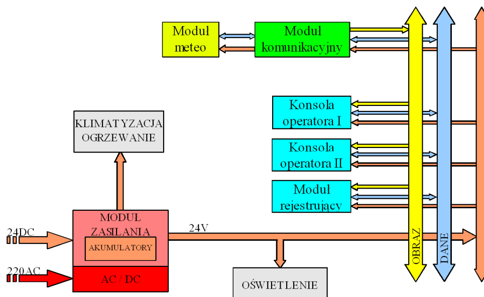
Rysunek 2.10. Schemat blokowy SKM
