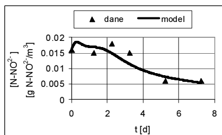
Rys. 20. Przebieg stężenia azotu azotynowego w czasie. Przekrój powyżej wylotu kolektora. Próbkę z osadem
