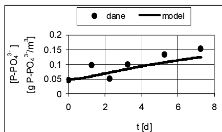
Rys. 22. Przebieg stężenia ortofosforanów w czasie. Przekrój powyżej wylotu kolektora. Próbkę z osadem
