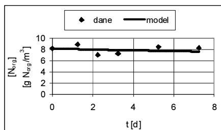
Rys. 18. Przebieg stężenia azotu organicznego w czasie. Przekrój powyżej wylotu kolektora. Próbkę z osadem
