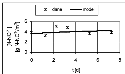
Rys. 21. Przebieg stężenia azotu azotanowego w czasie. Przekrój powyżej wylotu kolektora. Próbkę z osadem
