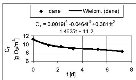
Rys. 16. Przebieg stężenia tlenu w czasie. Przekrój poniżej wylotu kolektora. Próbkę bez osadu, otwarta
