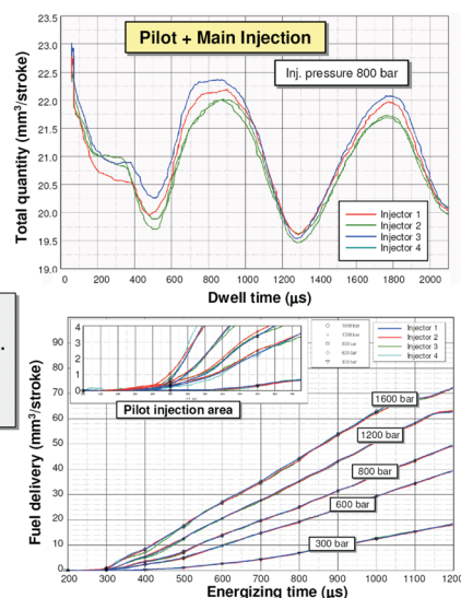
Rys. 10. Wtryskiwacz R. Bosch CRI2.2
