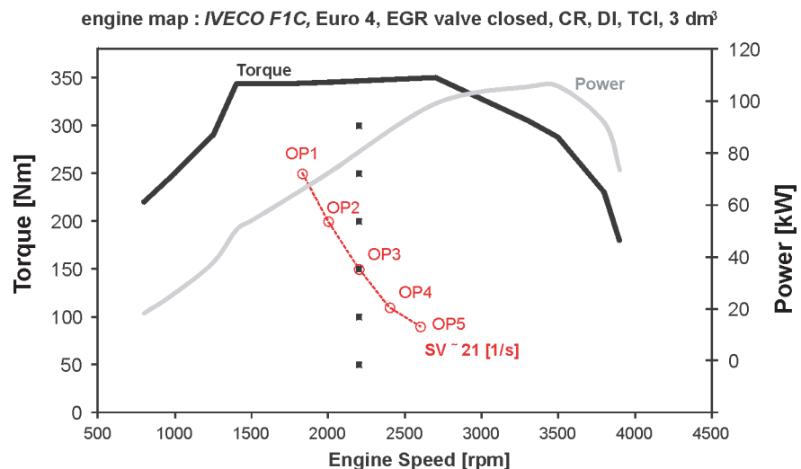
Fig. 3. Operating points in steptest and at SV = const on the Iveco engine Rys. 3. Punkty pomiarowe w teście stacjonarnym i przy SV = const na silniku Iveco
