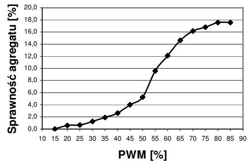
Rys. 4. Sprawność agregatu pompowego jako funkcja impulsu sterującego
