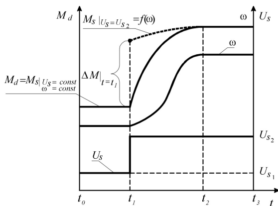
Rys. 3 Schemat procesu rozpędzania silnika [13]
