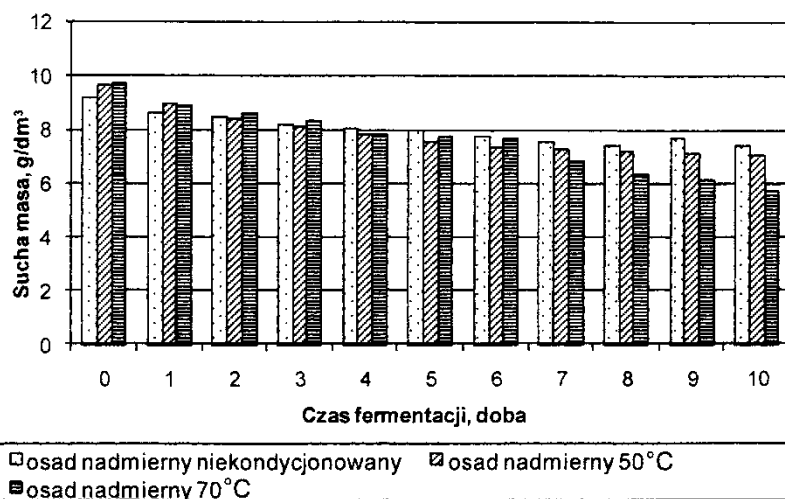
Rys. 3. Wpływ czasu fermentacji na suchą masę osadów nadmiernych kondycjonowanych termicznie
