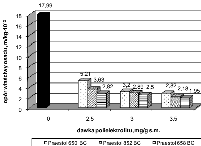
Rys. 3. Wpływ dawki polielektrolitu na opór właściwy osadu przefermentowanego
