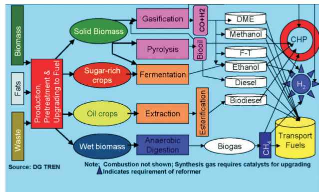
Rys. 23. Podstawowe procesy pozyskiwania paliw ze źródeł odnawialnych
