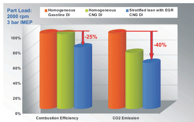
Rys. 12. Poprawa zużycia paliwa i emisji CO 2 w silniku zasilanym CNG w porównaniu do silnika konwencjonalnego Fig. 12. Fuel consumption and CO 2 emissions reduction in CNG Direct Injection in comparison with stoichiometric homogeneous charge engine
