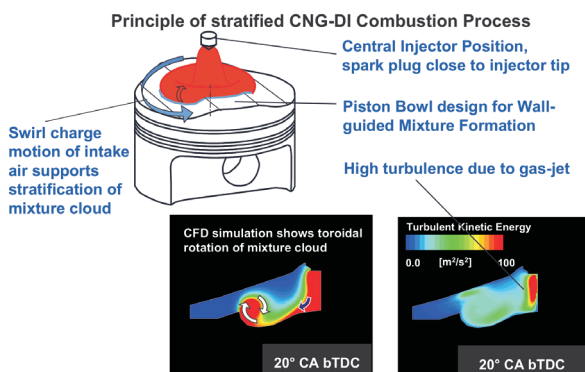
Rys. 10. Zasada działania systemu spalania z bezpośrednim wtryskiem gazu Fig. 10. Principle of stratified CNG-DI combustion process
