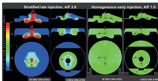
Rys. 11. Symulacja typu CFD (Computed Fluid Dynamic) tworzenie mieszanki w silniku z wtryskiem gazu przy pracy na mieszance uwarstwionej (rys. lewy) i mieszance jednorodnej (rys. prawy) Fig. 11. CFD simulation; mixture formation in the engine with stratified gas injection (on the left) and homogeneous gas injection (on the right)
