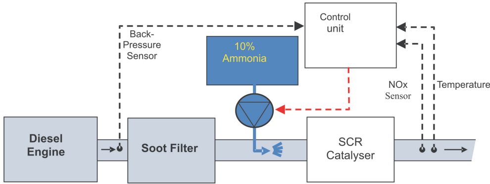
Rys. 29. Schemat układu wylotowego silnika wyposażonego w filtr cząstek stałych i katalizator deNOx z układem SCR Fig. 29. The structure of the engine exhaust system with PFS and DeNOx catalyst with SCR
