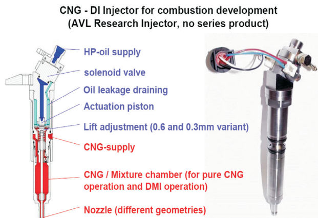
Rys. 9. Przekrój i widok wtryskiwacza do zasilania gazem CNG Fig. 9. The cross-section of the CNG injector
