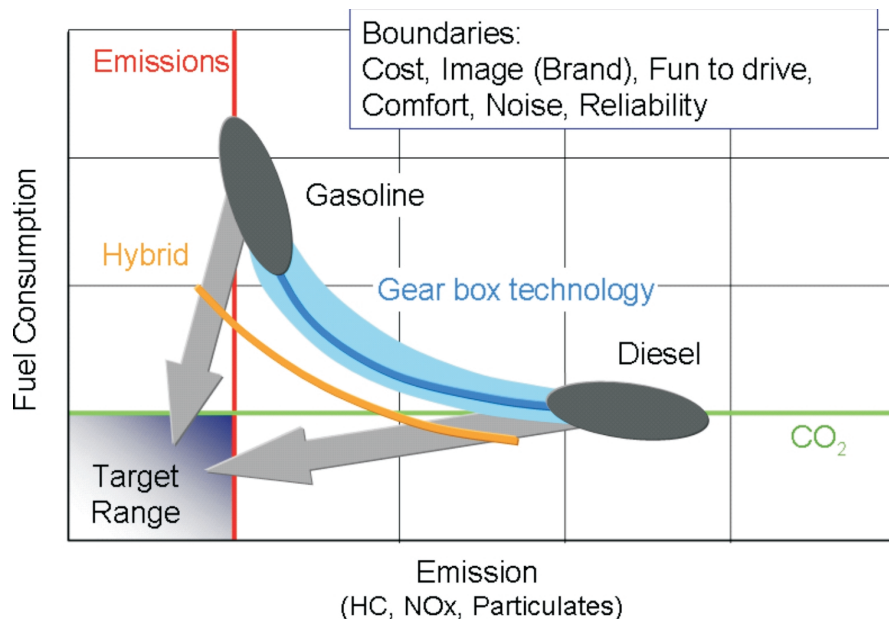
Rys. 3. Główne kierunki rozwoju napędów samochodów osobowych Fig. 3. Main PC powertrains development directions
