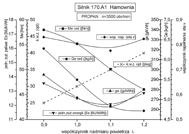
Rys. 11. Charakterystyka regulacyjna składu mieszanki \lambda silnika 170.A1, prędkość obrotowa wału korbowego silnika n = 3500 obr/min, pełne otwarcie przepustnicy, zasilanie wtryskowe propanem
