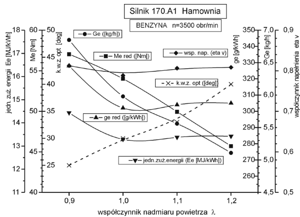
Rys. 8. Charakterystyka regulacyjna składu mieszanki \lambda silnika 170.A1, prędkość obrotowa wału korbowego silnika n = 3500 obr/min, pełne otwarcie przepustnicy, zasilanie wtryskowe benzyną
