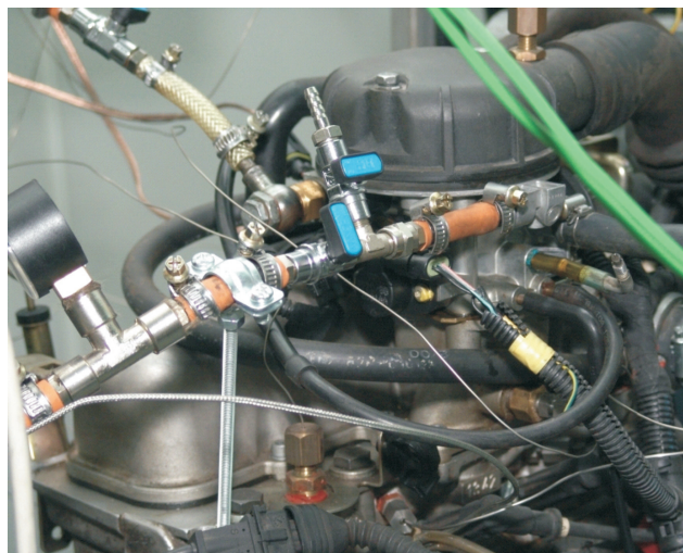
Kys. 6. Elementy układu zasilania silnika ciekłym gazem Fig. 6. Elements of the liquid gas feeding system
