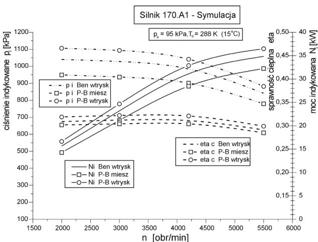
Rys. 1. Symulowana charakterystyka prędkościowa silnika 170.A1, ciśnienie w przewodzie dolotowym p_s = 95 kPa, temperatura otoczenia T_o = 288 K ( 15^\circ\text{C} ), zasilanie mieszalnikowe propanem-butanem, wtryskowe benzyną lub propanem-butanem, skład mieszaniny propanu i butanu 50/50
