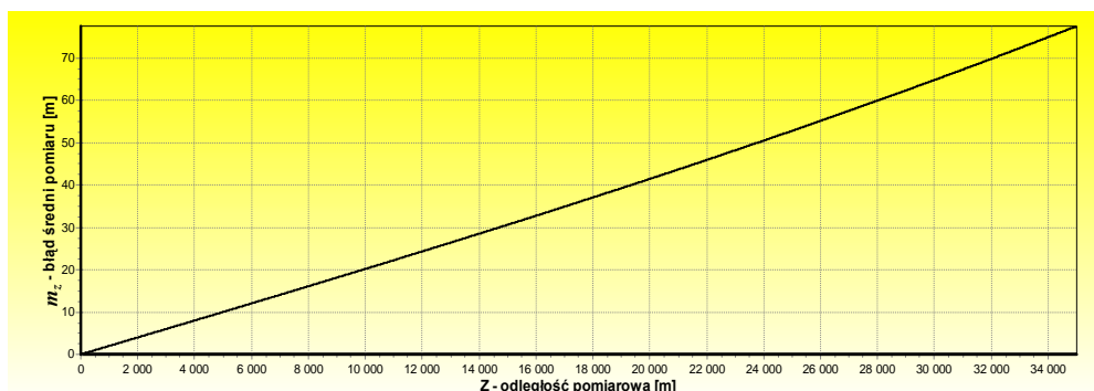
Rys. 4. Wykres zmiany wartości błęd średni m_z pomiaru wykonanego kamerą Rolleiflex 6008
