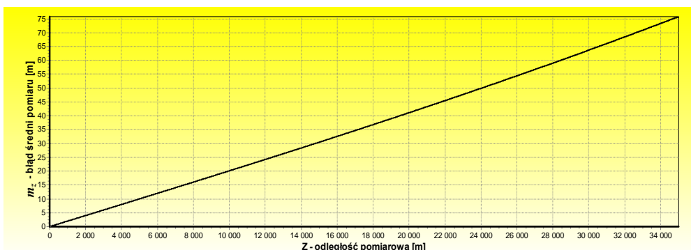
Rys. 5. Wykres zmiany wartości błędu średniego m_z pomiaru wykonanego kamerą Sony \alpha 900 F4-5.6 G SSM
