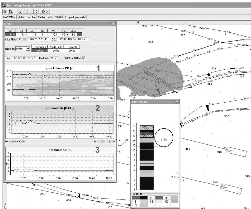
Fig. 4. Elevation of bucket wheel and qualitative parameters of the coal (left part of the figure) Rys. 4. Podwyższenie koła czepakowego i parametrów jakościowych węgla (lewa część rysunku)
