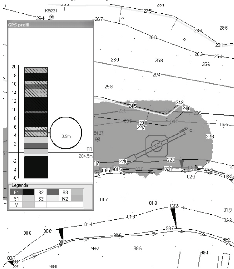
Fig. 3. The position of the bucket wheel excavator in real time (map and profile) Rys. 3. Pozycja tyżki koparki kołowej w czasie rzeczywistym (mapa i profil)
