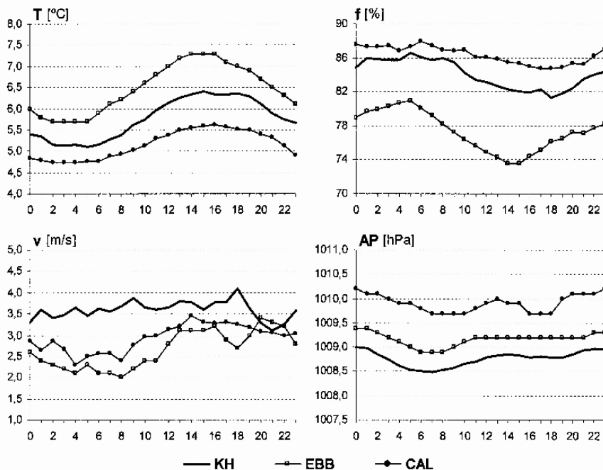
Ryc. 3. Średnie przebiegi dobowe temperatury powietrza (T), wilgotności względnej (f), prędkości wiatru na 2m n.p.t. (v) oraz ciśnienia atmosferycznego na poziomie morza (AP) na stacjach: KH, EBB i CAL w okresie 21.07–31.08.2005 r.
