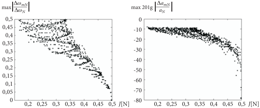
Rys. 9. Statystyki maksymalnego błędu estymacji pulsacji (19a) (po lewej) i maksymalnego błędu estymacji amplitud (19b) (po prawej)
