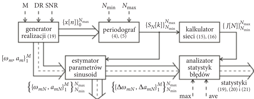
Rys. 1. Schemat eksperymentu numerycznego
