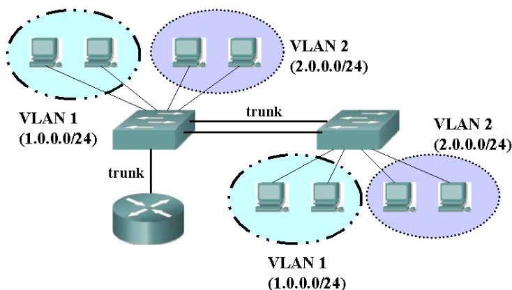
Rys. 13. "Jednoręki" router łączący sieci VLAN
