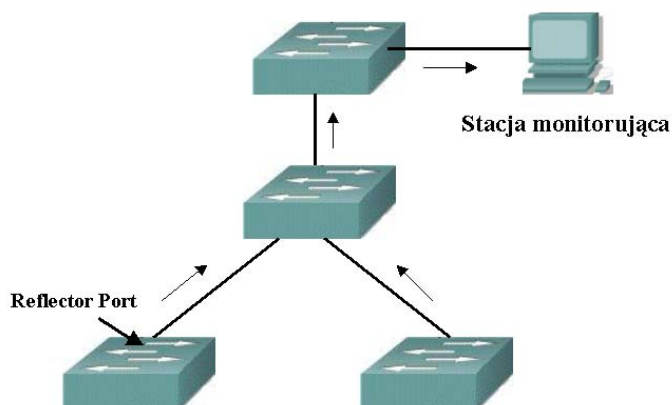
Rys. 12. Sesja RSPAN w środowisku kaskadowo połączonych przełączników
