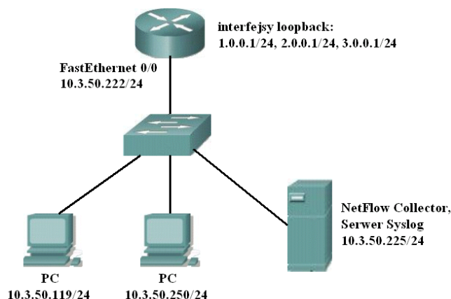
Rys. 2. Proste środowisko badawcze z routerem serii 2600 i NetFlow Collectorem
