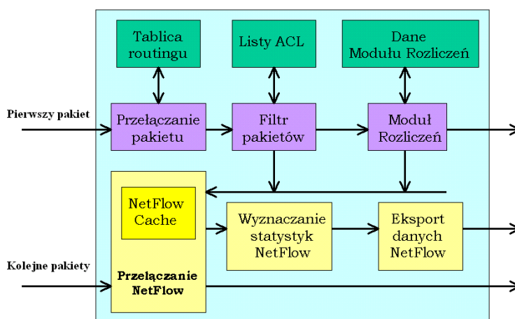
Rys. 1. Obsługa pakietów przez router z uruchomionym trybem przełączania NetFlow [3]
