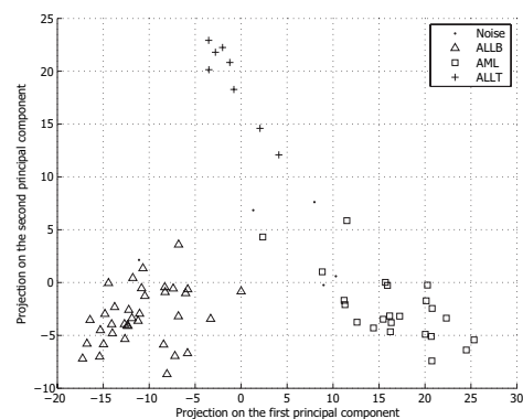
(d) DBSCAN
