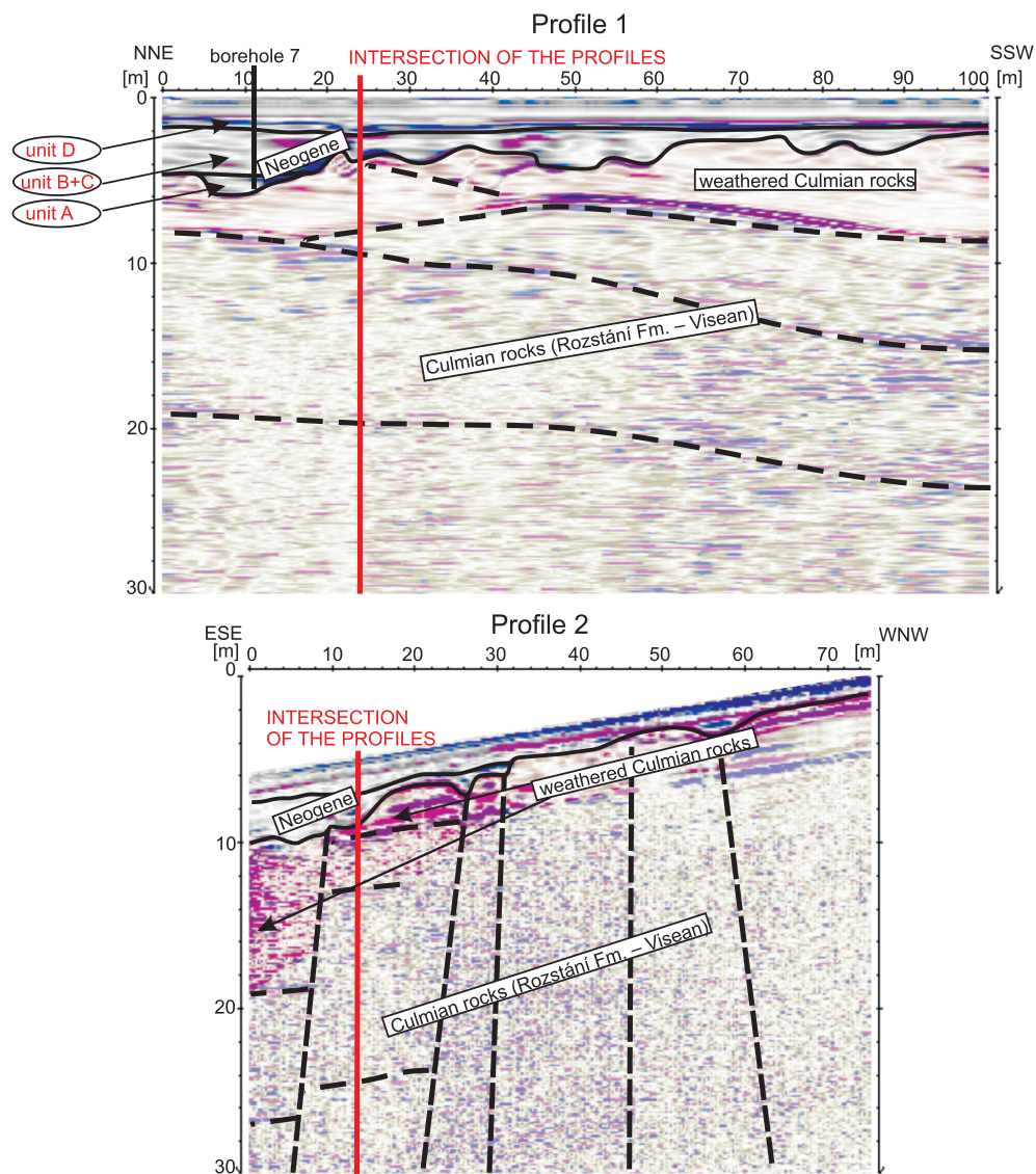
Fig. 3. Interpretation of georadar profiles at the Přemyslovice locality
