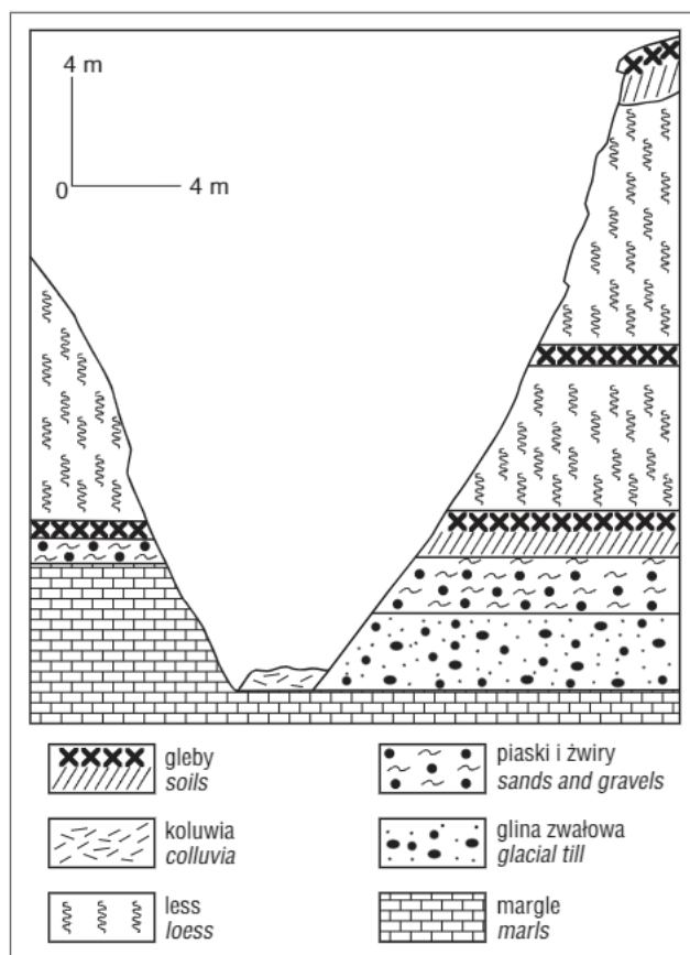
Ryc. 3. Budowa geologiczna zboczy wąwozu Chałajowy Dół (za Gardzielem i in., 2006)
