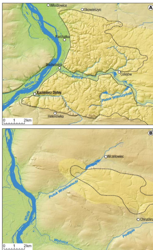
Ryc. 2. Różnorodność rzeźby lessowej zachodniej części Wyżyny Lubelskiej. A – silnie rozcięta zachodnia część Płaskowyżu Nałęczowskiego (regiony wąwozowe 1 i 2 na ryc. 1); B – słabo rozcięta zachodnia część Wzniesień Urzędowskich z osobliwymi formami akumulacji lessowej (region wąwozowy 5 na ryc. 1)
