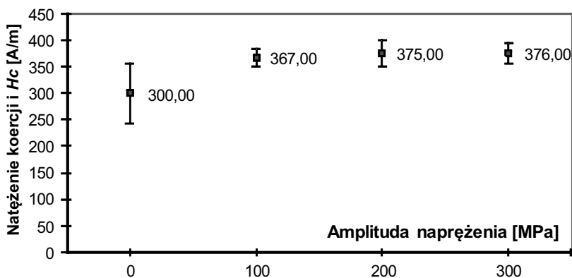
Rys. 9. Wynik analizy zmian natężenia koercji H_c w funkcji amplitudy naprężenia
