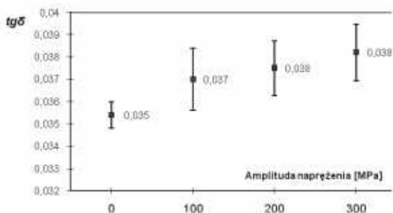
Rys. 12. Zmiany tangensa kąta strat ( \tan \delta ) w zależności od amplitudy naprężeń
