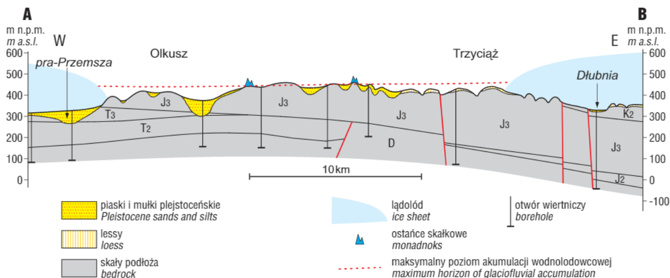
Ryc. 2. Przekrój geologiczny A–B (zob. ryc. 3), ilustrujący strukturalne założenia „Jurajskiej Oazy Śródlodowej”. Litostratygrafia: K 2 – margle kredy górnej, J 3 – wapień jury górnej, T 3 – ilowce i mułowce triasu górnego, T 2 – wapień i dolomity triasu środkowego, D – wapień dewonu
