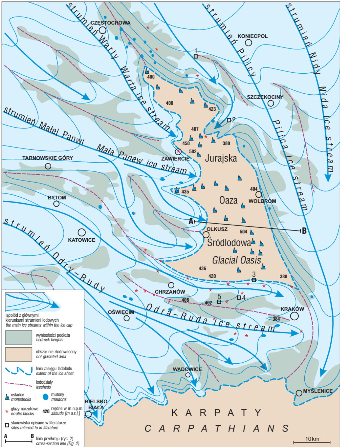
Ryc. 3. Paleogeografia Wyżyny Śląsko-Krakowskiej podczas zlodowacenia sanu I. Odślonięcia opisane w literaturze: 1 – Julianka (Różycki, 1982b), 2 – Pradła (Semil, 1982), 3 – Dolina Kobylańska (Walczak, 1956), 4 – Nielepice (Zareczny, 1956), 5 – Rudna (Rutkowski i in., 1998)
