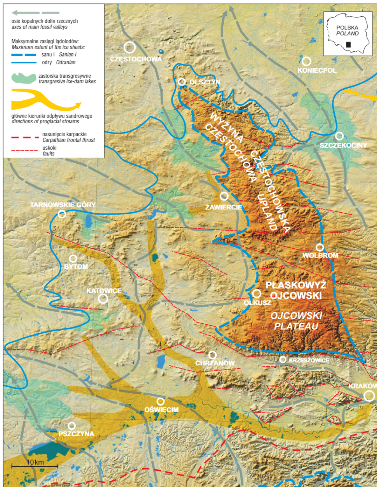
Ryc. 1. Główne elementy paleogeografii plejstoceńskiej Wyżyny Śląsko-Krakowskiej na tle mapy cyfrowej rzeźby terenu (DEM)
