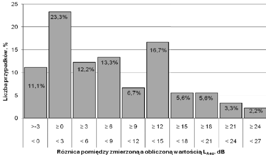
Rys. 2. Rozkład statystyczny różnic pomiędzy mierzonymi i obliczonymi poziomami dźwięku A pod 180 czasami nauszników przeciwbalansowych.
