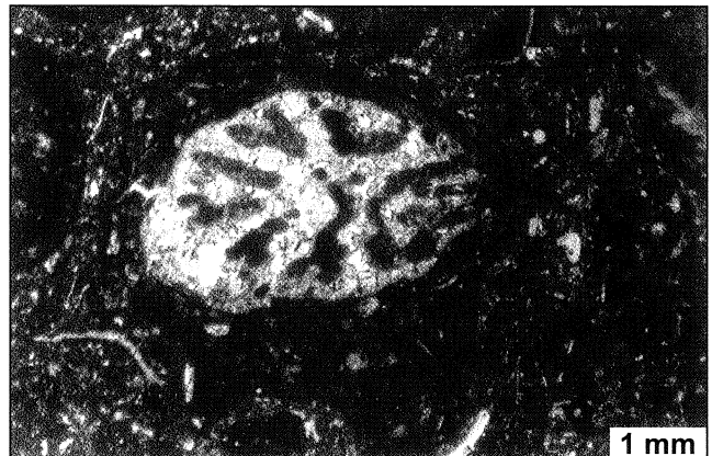
Fig. 13. Floatstone – wackestone with scleractinian coral (fragment of colony? pers. commun. E. Morycowa, B. Kołodziej, 2001); Księża Hill
