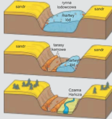
Rys. 15. Schemat powstania doliny Czarnej Hańczy na odcinku Sobolewo–ujście do jez. Wigry (K. Pochocka-Szwarc, M. Krzeczynska)
