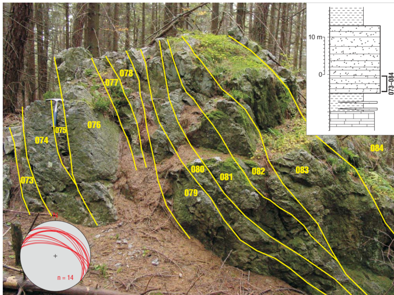
Ryc. 5. Profil 2 – część spagowa: piaskowce kwarcytowe. 073-084 numer warstwy, diagram w dolnej części: projekcja stereograficzna położenia warstw, dolna półkula, 14 pomiarów. Objasnienia szrafur na ryc. 9. Fot. R. Zabielski
