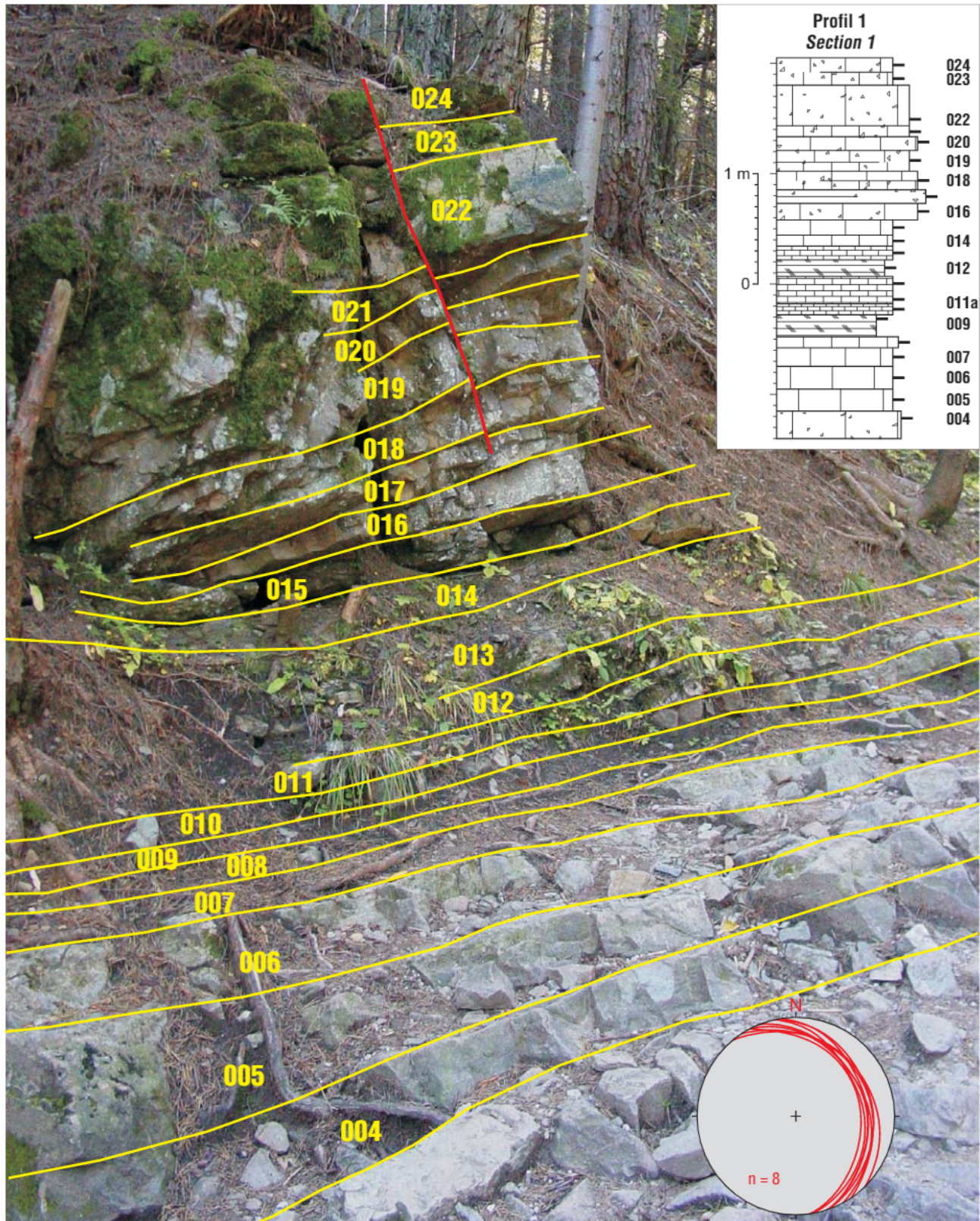
Ryc. 8. Profil 1. Piaskowce wapienne. 004–024 numery warstw, diagram w dolnej części: projekcja stereograficzna położenia warstw – dolna półkula, 8 pomiarów. Fot. R. Zabielski. Objaśnienia szrafur na ryc. 9
