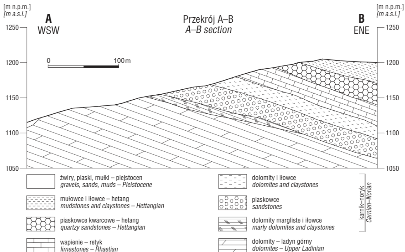
Ryc. 3. Przekrój A-B. Profil litologiczny wzdłuż ścieżki Kuźnice–Nosal. Objaśnienia symboli na ryc. 1 (uwaga: szrafury w obrębie wydzielen nie są współkształtne do uławiczenia)
