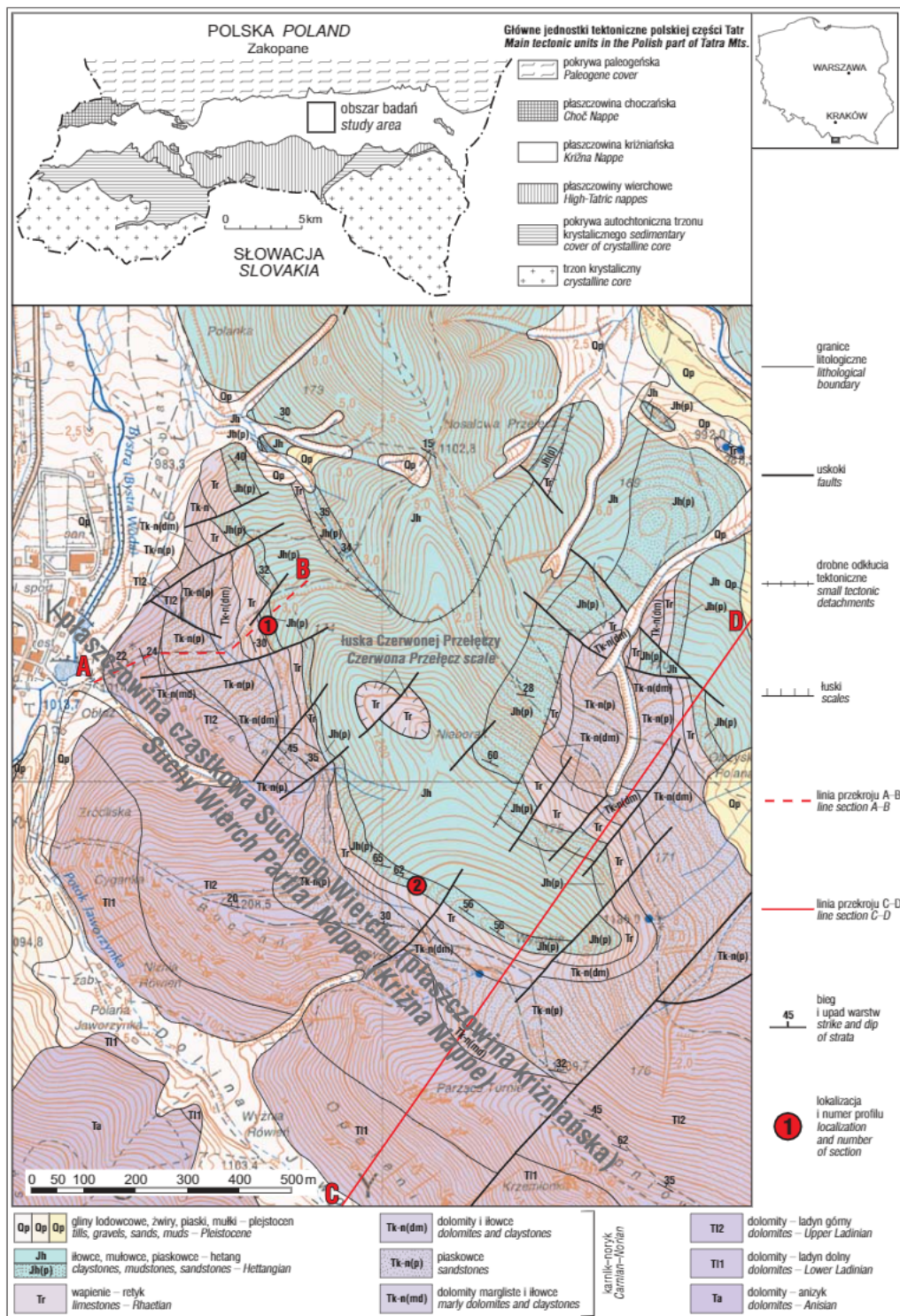
Ryc. 1. Obszar badań – fragment Szczegółowej Mapy Geologicznej Tatr w skali 1 : 10 000 w nowej edycji (arkusz Zakopane – Południe). Ta – dolomity (anizyk); Tl1 – dolomity (lądyn dolny); Tl2 – dolomity (lądyn górny); Tk-n(md) – dolomity margliste oraz łupki mułowcowo-ilaste (kajper dolny); Tk-n(p) – piaskowce kwarcytowe z przewarstwieniami łupków mułowcowo-ilastych (kajper środkowy); Tk-n(dm) – łupki mułowcowo-ilaste z przewarstwieniami dolomitów (kajper górny); Tr – wapienie organogeniczne i organodetrytyczne z wkładkami łupków i z piaskowcami wapienistymi w części górnej (formacja fatrzańska – retyk); Jh(p) – piaskowce kwarcytowe ławicowe (hetang), Jh – łupki ilasto-mułowcowe z przewarstwieniami wapieni (formacja z Kopiańca – hetang); Qp – muł, piasek, żwir, glina lodowcowa (plejstocen nierozdzielny)
