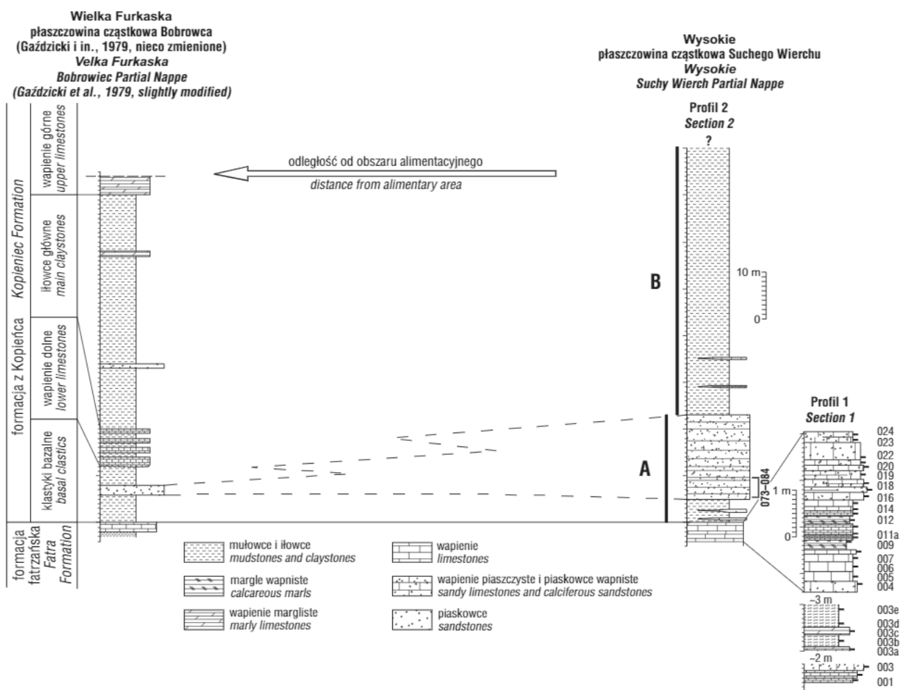
Ryc. 9. Korelacja profili litofacjalnych dolnej części utworów formacji z Kopieńca w płaszczowinach cząstkowych Suchego Wierchu i Bobrowca
