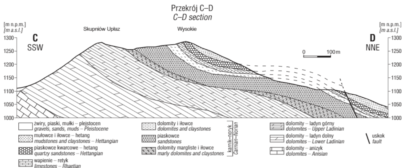
Ryc. 4. Przekrój C–D. Objasnienia symboli jak na ryc. 1 ( uwaga: szrafury w obrębie wydzieleni nie są współkształtne do uławicenia ) Fig. 4. Section C–D. For explanation see Fig. 1. ( attention: hatchings are not parallel to stratification )
