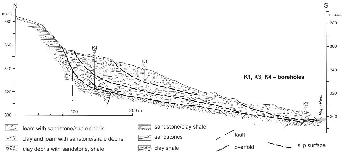
Fig. 2. Longitudinal section of the landslide (after A. Wójcik in: Zabuski et al. , 2004)
