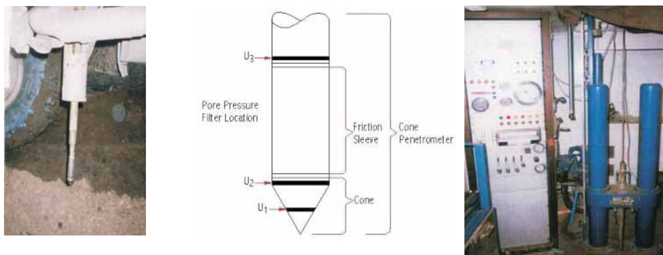
Fig. 5. Piezocone test equipments (A P Van den Berg penetrometer Hysson 200)
