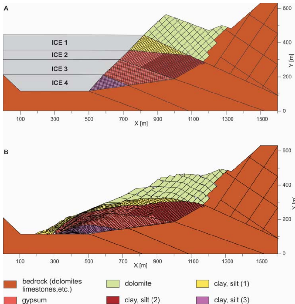
Fig. 7. Development of the Passo della Morte landslide
